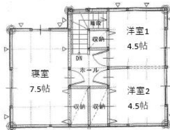
2階 平面図
