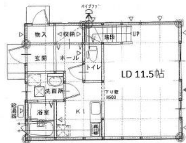
1階 平面図
